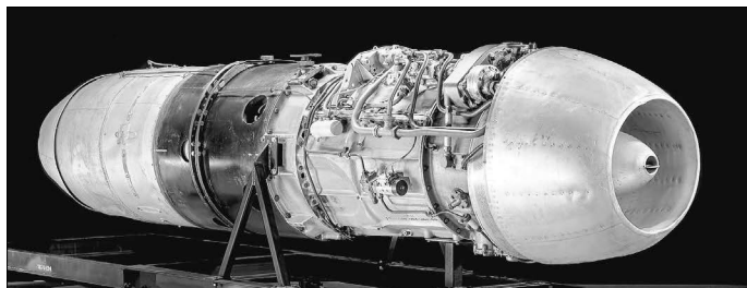
JUMO-004 Triebwerk der Me 262
