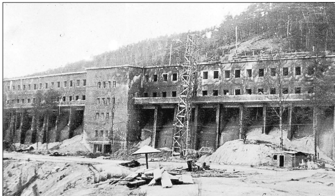
Bunker 0, Stützpfeiler an der Außenseite für das aufgesetzte Betriebsgebäude
