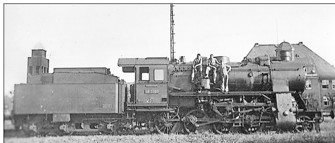
Eine der zwei Lokomotiven
