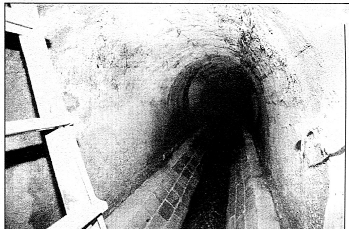
Ein aus Naturstein gemauerter Durchlass führt das Wasser des Baches unter dem Else-Härtel-Weg bis zur Saale. Der optische Eindruck dieses Bauwerkes ist gut, so dass nicht mit größeren Sanierungsarbeiten gerechnet werden muss.
