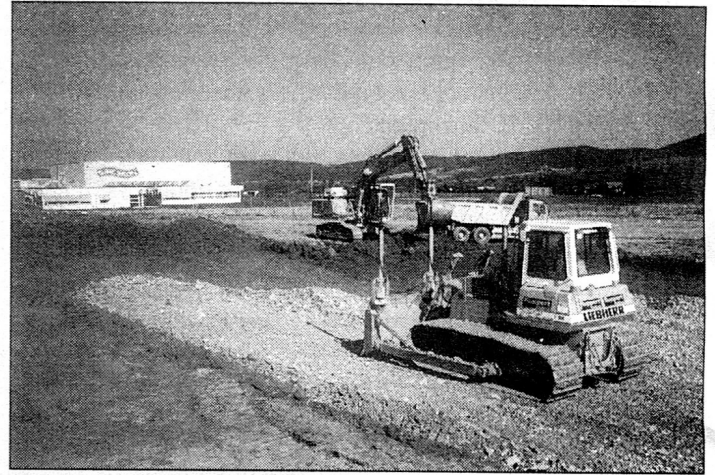
Schwere Bautechnik beim Herstellen des Planums für das Industriegebäude.
