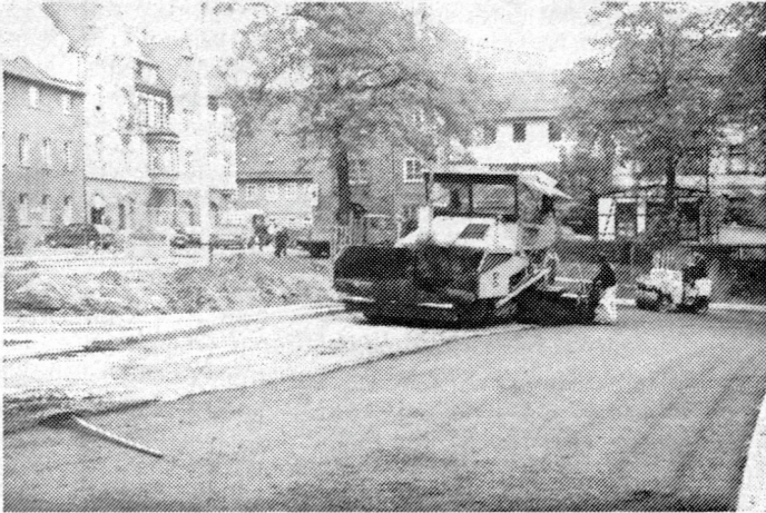
Einbau der Tragschicht im Bereich der LIO 62
