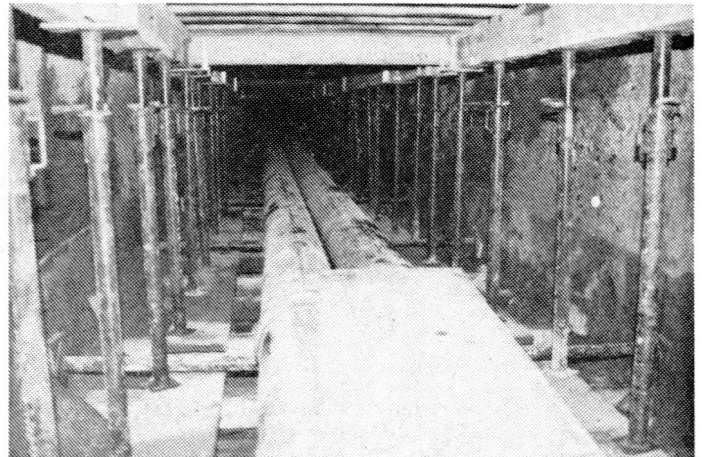
Schalungsunterkonstruktion und provisorische Wasserführung in Plasterohren
